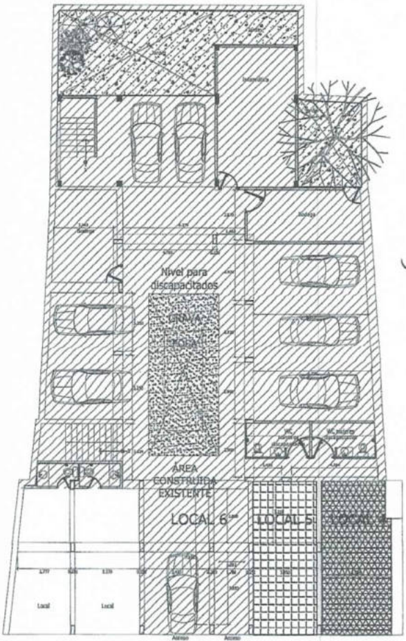
PLANTA BAJA
